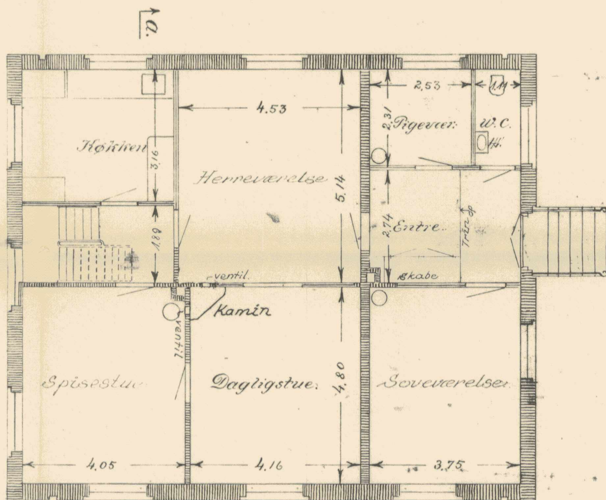
Stueplan.
