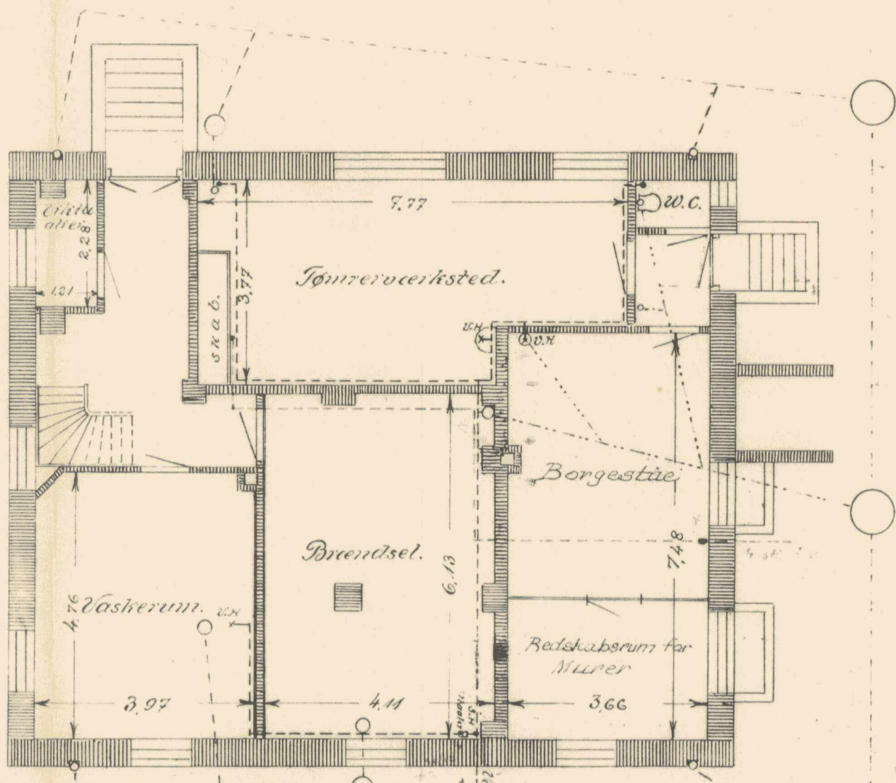
Kelderplan.
