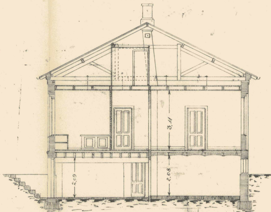
Tværsnit a-b.
