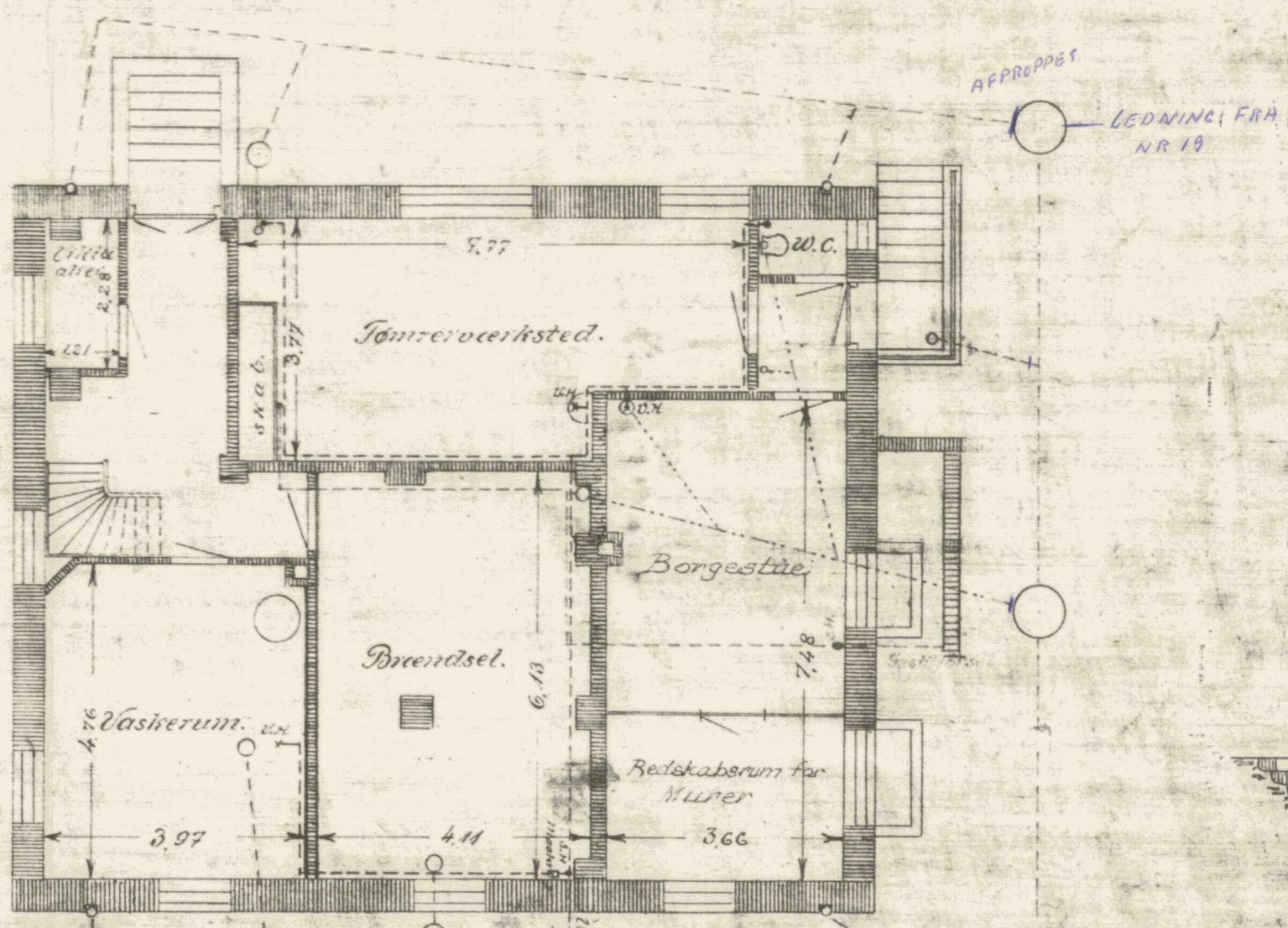
Kælderplan.
