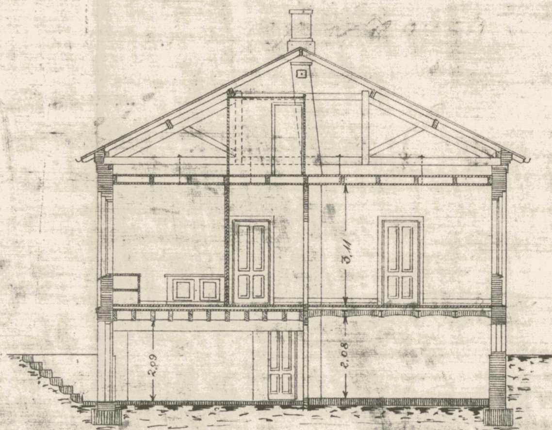
Tværsnit a-b.
