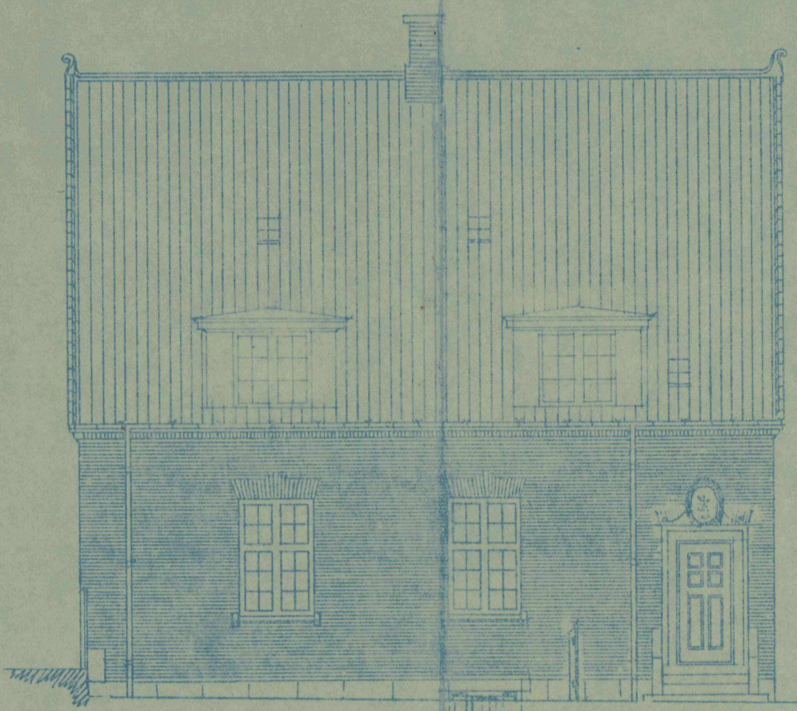
MOD HOVEDBYGNING
